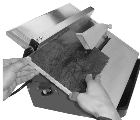
Figure I: Bevel Cuts
